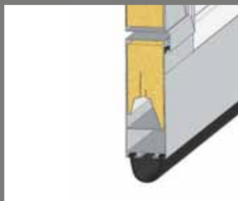
Standardní práh výška prahu 140+20 mm
