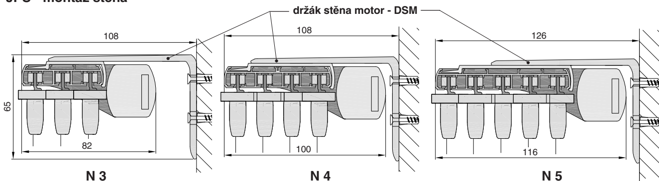
JPS - montáž stěna - motor
