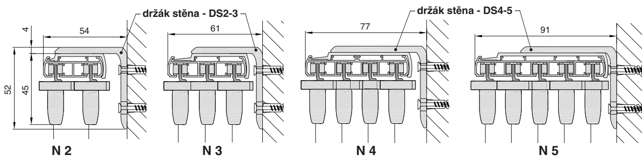
JPS - montáž stěna
