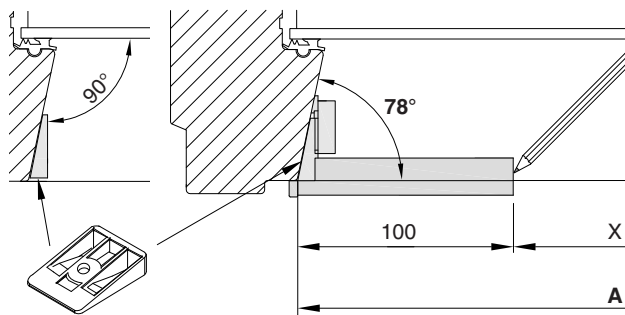
Podložka 78°
