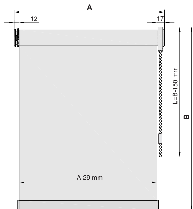
APOLLO - řetízek
