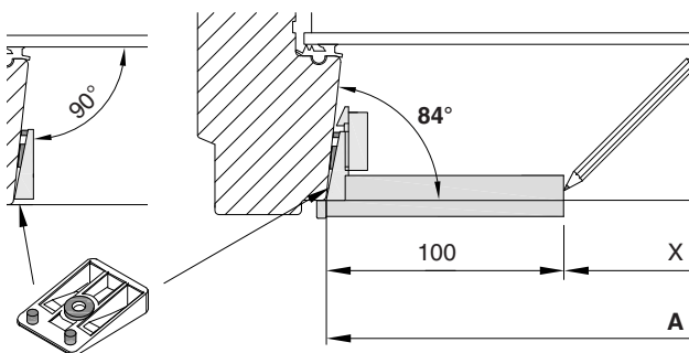
Podložka 84°
