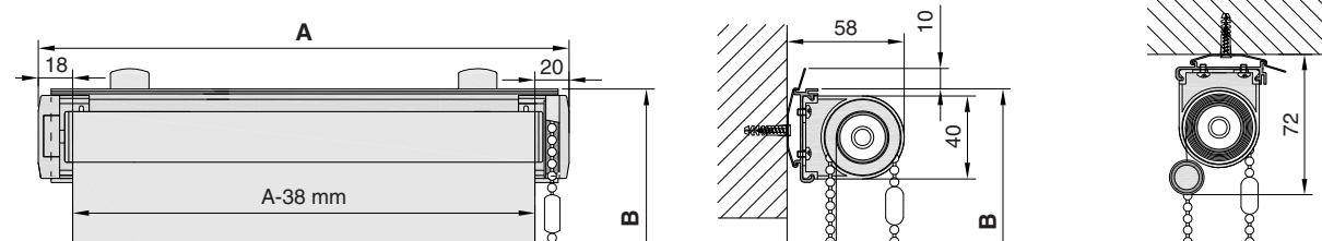
MODULA 25 - P (s montážním Profilem)
