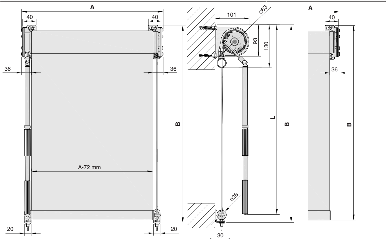
V63 - klika s vedením
