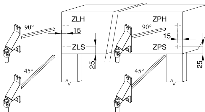
Zadní vývod průchodky kliky
