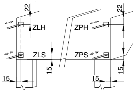
Zadní vývod průchodky kliky
