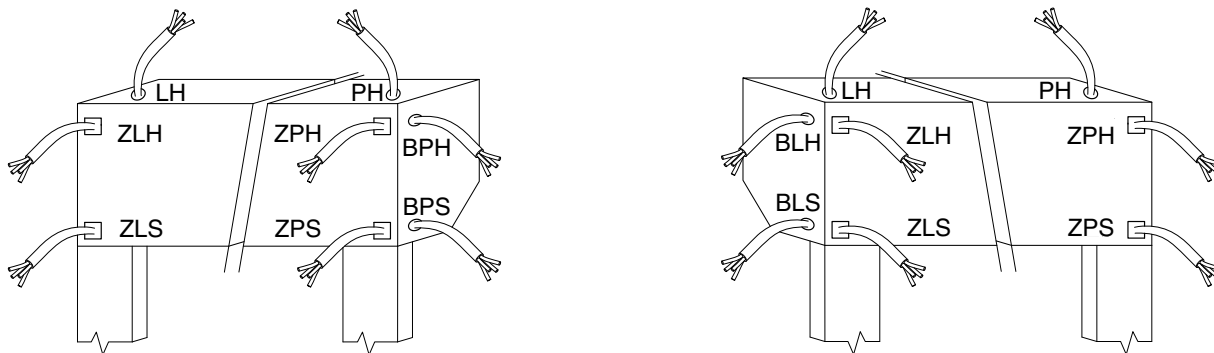
Zadní vývod kabelu u motorického ovládání
