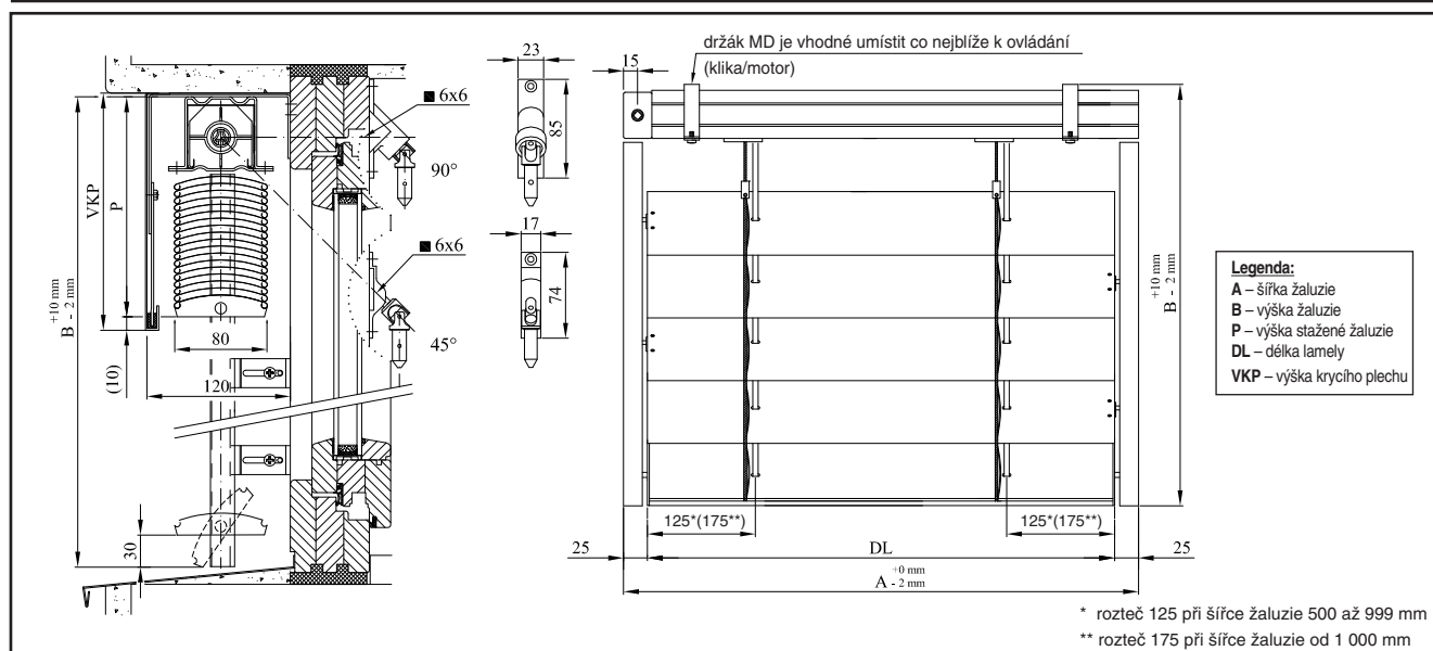
C-80 - Vedení v lištách
