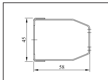
DZ - Držák pro montáž na stěnu
