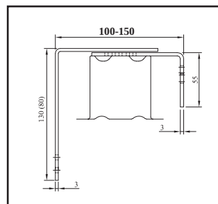
DK 5 - Držák krycího plechu posuvný
