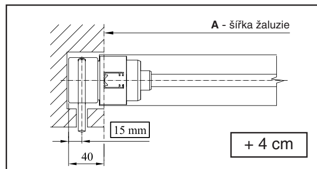
Příklad kladného posunutí převodovky + 4 cm
