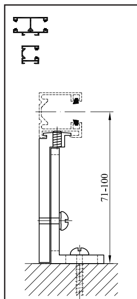
K 2 - Konzola vodící lišty
