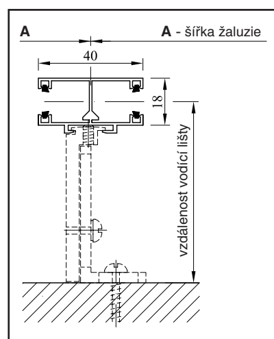
VL 3 - Vodící lišta dvojitá
