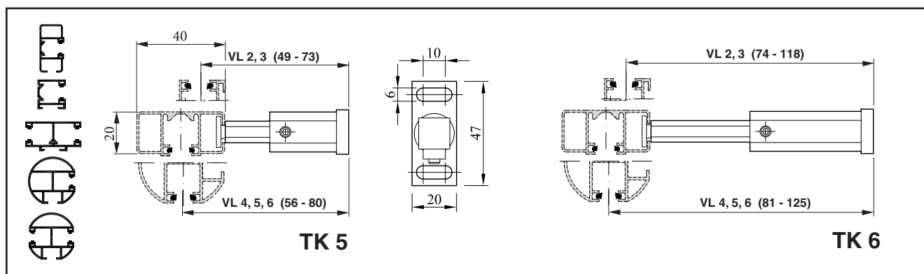
TK 5, TK 6 - Teleskopická konzola vodicí lišty
