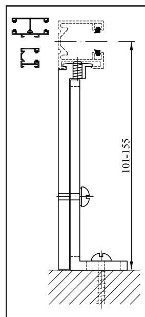
K 3 - Konzola vodící lišty
