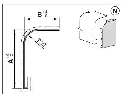
KP 1e L = A + B
