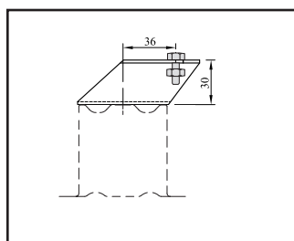
Z - Držák do překladu Heluz 165
