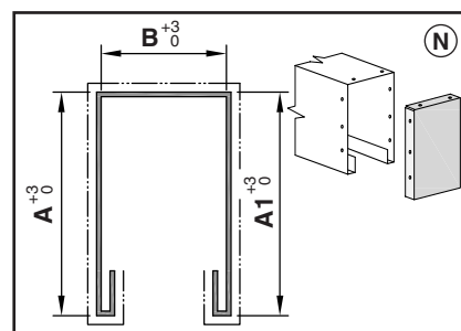
KP 3a L = A + B + A1
