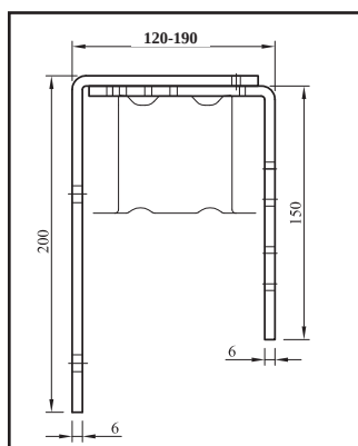
PP - Držák podomítkový posuvný
