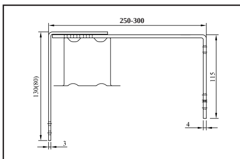
DK 8b - Držák krycího plechu posuvný prodloužený
