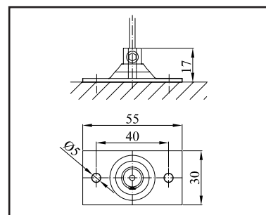
DL 4 - Držák lanka pro kotvení do podlahy
