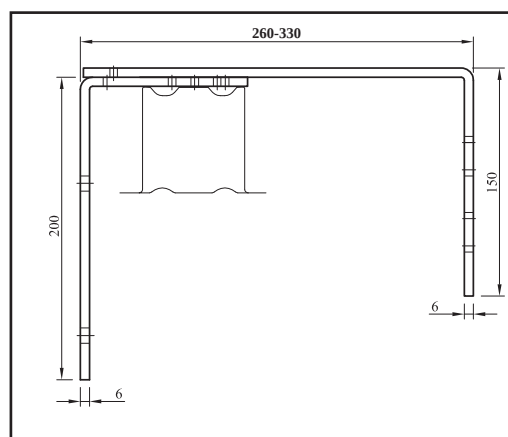
PPF 3 - Držák podomítkový fasádní posuvný
