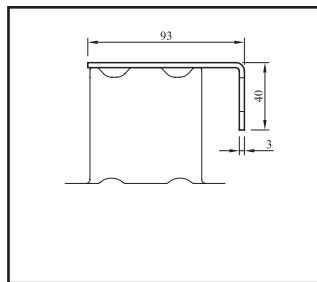
MD 2a - Montážní držák na rám
