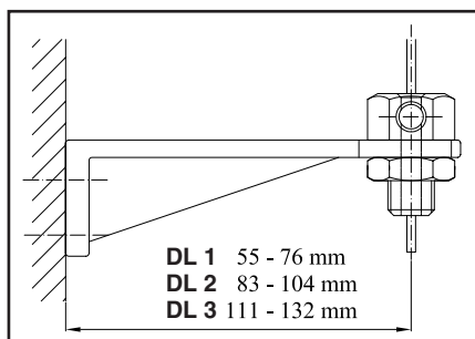
DL 1, DL 2, DL 3 - Držák lanka
