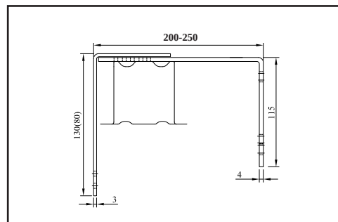
DK 7b - Držák krycího plechu posuvný prodloužený
