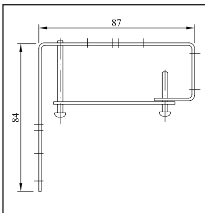
DKP - Držák pro montáž krycího plechu
