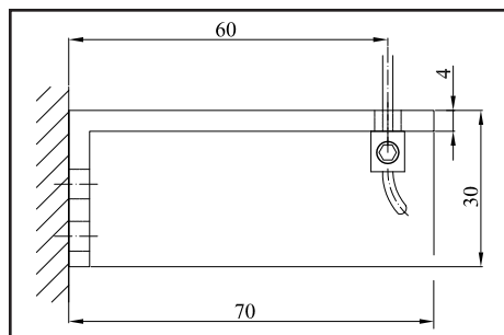
DL - Držák lanka standard
