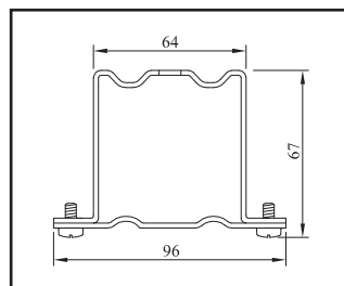
MD 1 - Montážní držák standard
