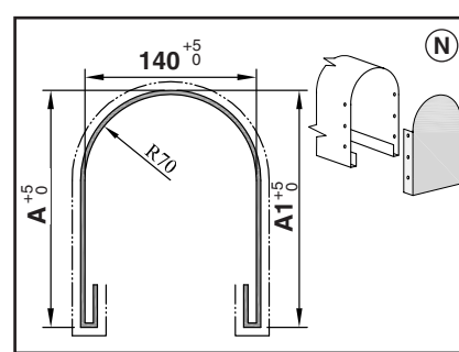
KP 3e L = A + A1 + 140
