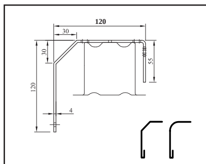
DK 3a - Držák krycího plechu zkosený pro C-80, Z-70, F-80
