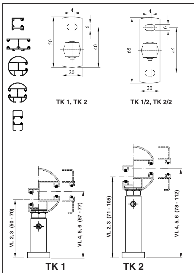
TK 1, TK1/2, TK2, TK 2/2 - Teleskopická konzola vodicí lišty
