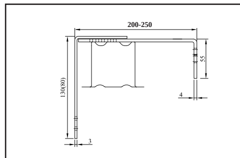
DK 7 - Držák krycího plechu posuvný
