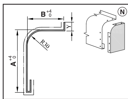
KP 2e L = A + B + Y
