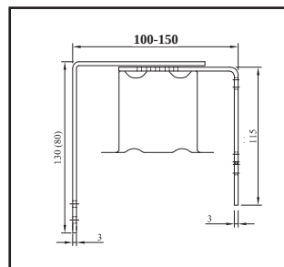
DK 5b - Držák krycího plechu posuvný prodloužený
