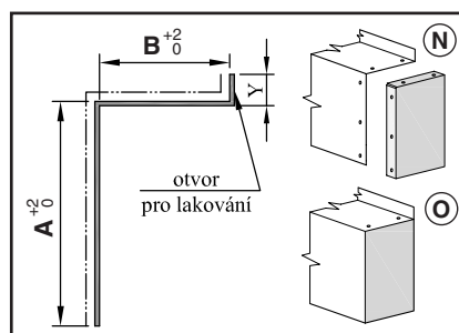
KP 2b L = A + B + Y
