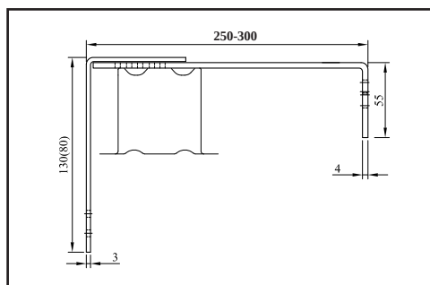
DK 8 - Držák krycího plechu posuvný
