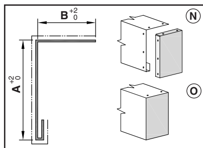
KP 1a L = A + B
