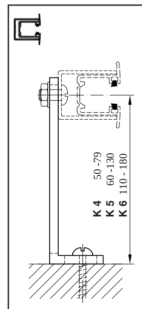
K 4, K 5, K 6 - Konzola pro zápuštěné pouzdro ZP
