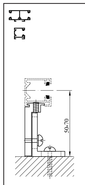
K 1 - Konzola vodící lišty
