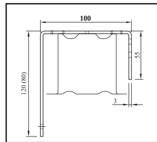
DK 2 - Držák krycího plechu pro Z-70, EXT-50 H
