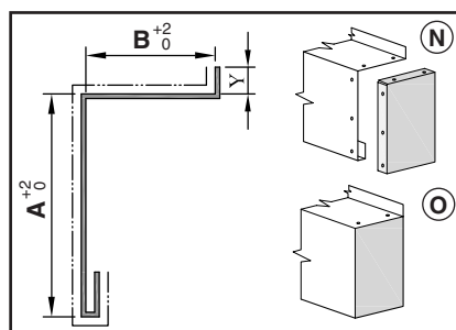
KP 2a L = A + B + Y
