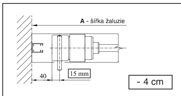
Příklad záporného posunutí převodovky - 4 cm
