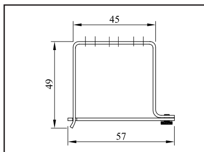
DS - Držák pro montáž na strop
