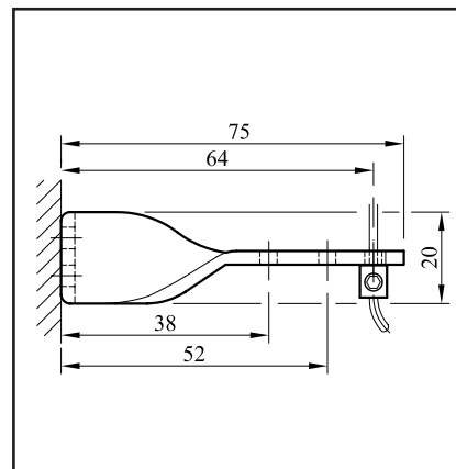
DL 5 - Držák lanka
