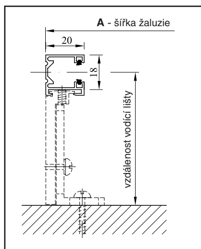
VL 2 - Vodící lišta na konzolu
