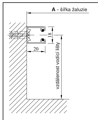
VL 1 - Vodící lišta do ostění
