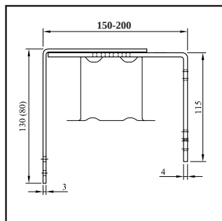
DK 6b - Držák krycího plechu posuvný prodloužený
