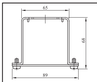
MD 1a - Montážní držák nerez
