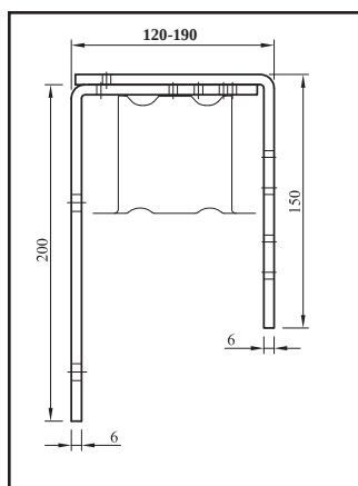
PPF 1 - Držák podomítkový fasádní posuvný
