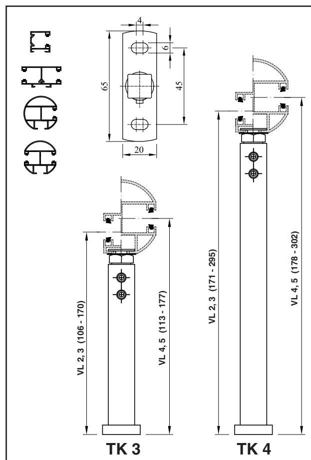
TK 3, TK 4 - Teleskopická konzola vodicí lišty
