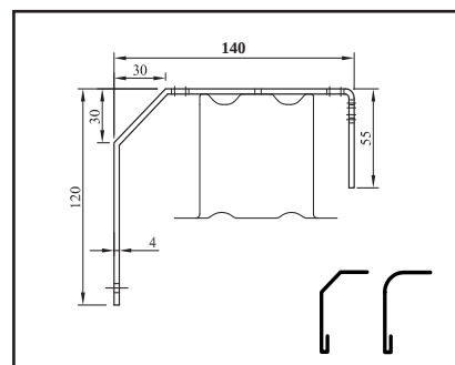
DK 4a - Držák krycího plechu zkosený pro Z-90
