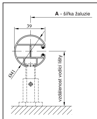
VL 4 - Vodící lišta kulatá
