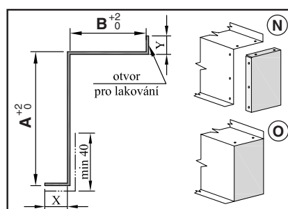
KP 2c L = X + A + B + Y
