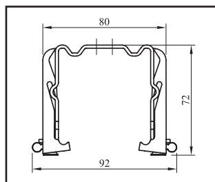
MD 1b - Montážní držák pružinový
