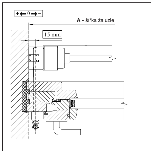
Standardní umístění převodovky
