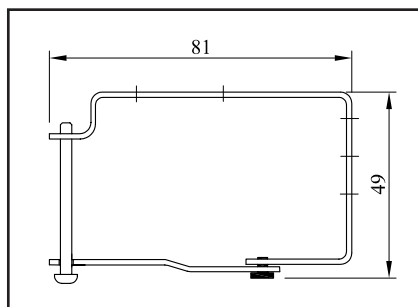
DU - Držák univerzální
