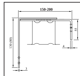
DK 6 - Držák krycího plechu posuvný
