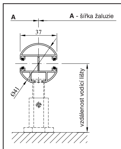
VL 5 - Vodící lišta kulatá dvojitá
