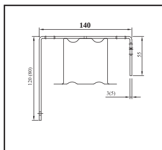
DK 4 - Držák krycího plechu pro Z-90
