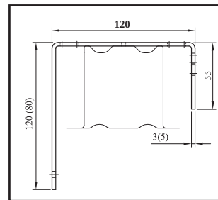
DK 3 - Držák krycího plechu pro C-80, Z-70, F-80
