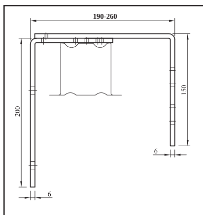
PPF 2 - Držák podomítkový fasádní posuvný
