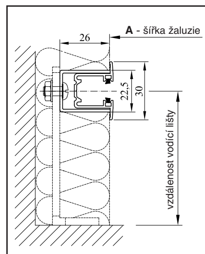
VL 7 - Vodící lišta zapuštěná se zápuštěným pouzdrům ZP
