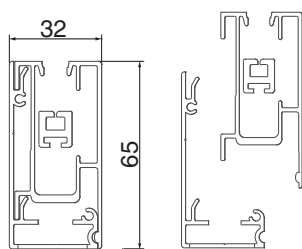
Vodicí lišta
