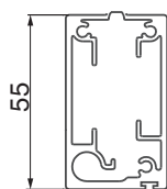
Spodní profil
